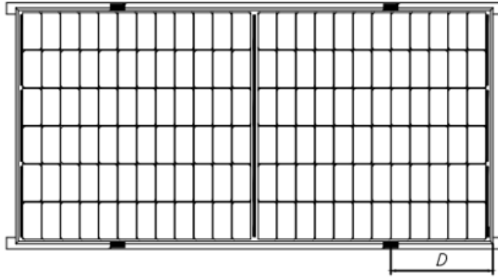
Fig. c Montageschienen verlaufen parallel zur langen Rahmenseite
