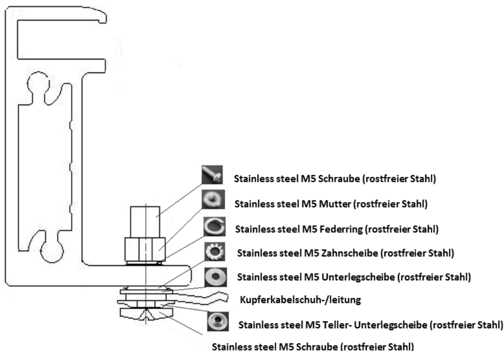
Fig h Erdung des Aluminiumrahmens mit einer Kupferleitung
