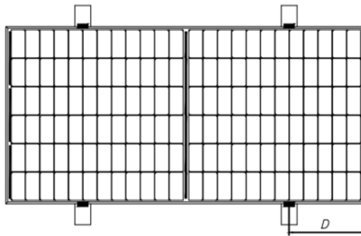
Fig. d Montageschienen verlaufen senkrecht zur langen Rahmenseite
